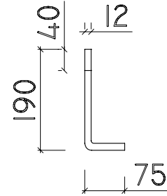
DETALLE PERNO
