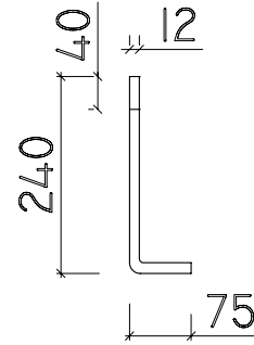
DETALLE PERNO
